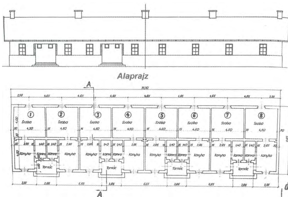
Ózd, az ún. Újhétes telep összképe, az egyik ház homlokzatai és alaprajza, 1940-1942
